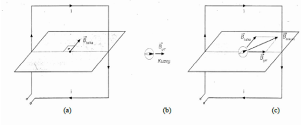
Şekil 4 Manyetik alan yönünün deney düzeneğinde gösterimi
