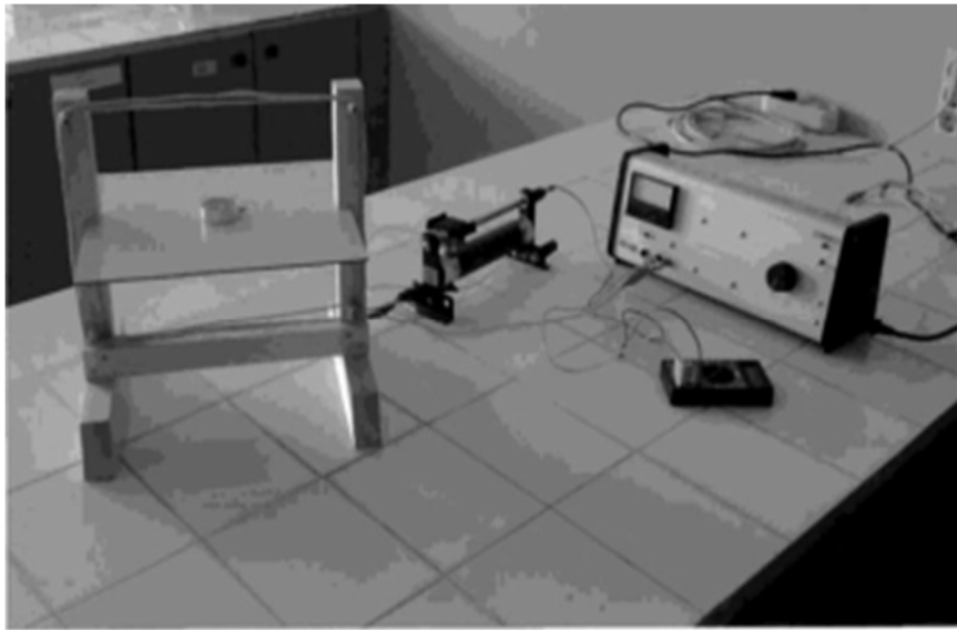
Şekil 3 manyetik alan deney düzeneği
