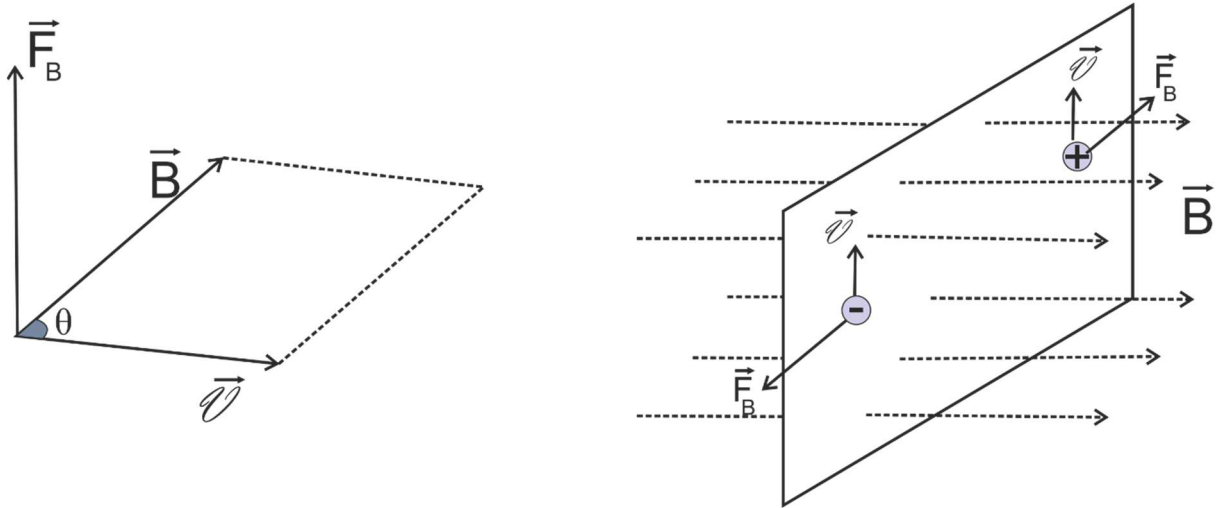
Şekil 1 Düzgün bir manyetik alanda hareket eden yüklü parçacığa etkiyen kuvvet
