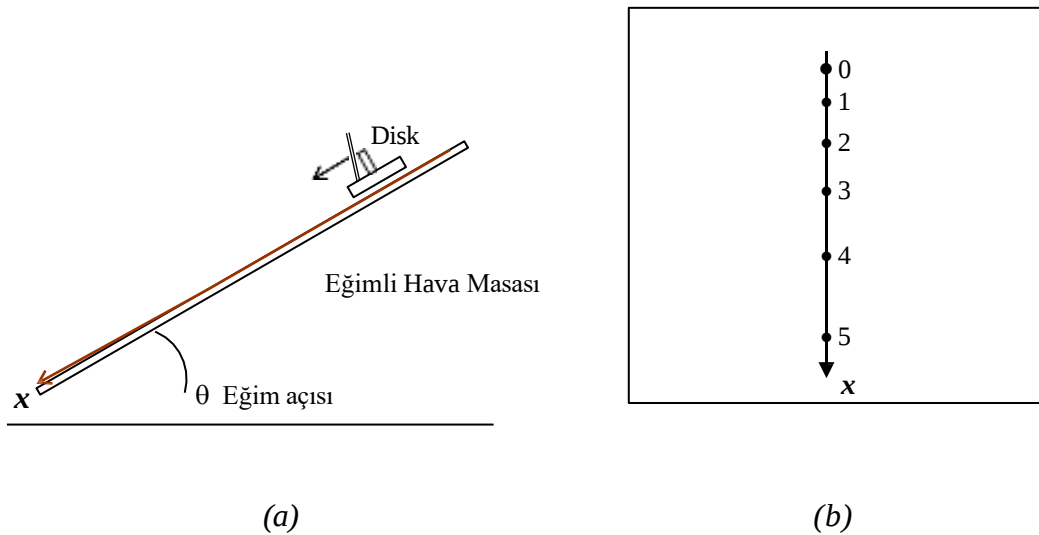
Şekil 1. (a) Eğimli bir hava masasında aşağı doğru hareket eden bir disk için deneysel kurulum.
