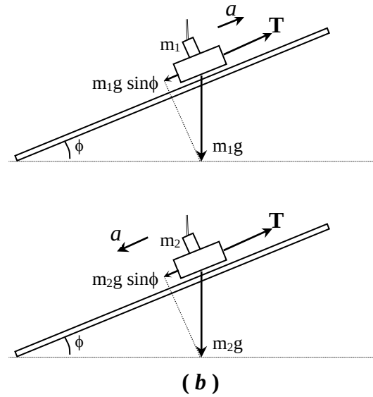
Şekil 2: Eğimli bir Hava Masasının üzerinde bir Atwood Makinasının deneysel kurulumu.
