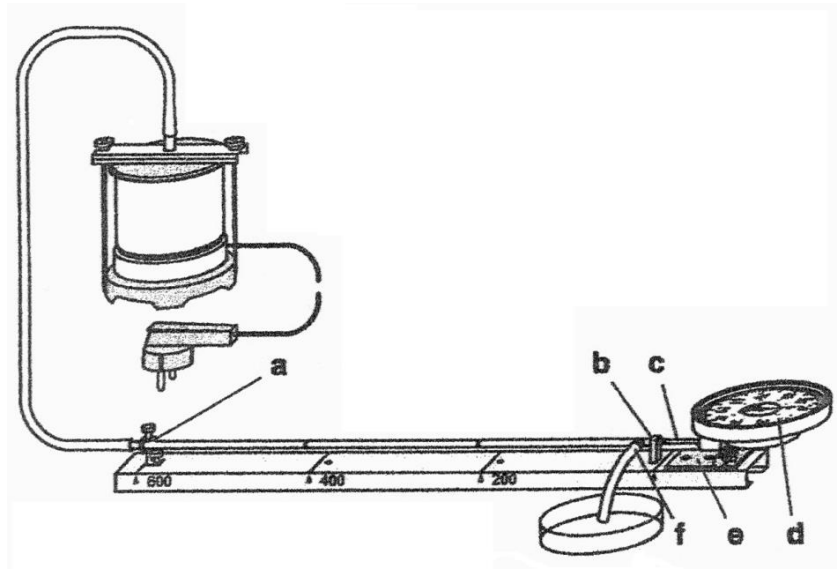
Şekil 1. Katıların genleşme katsayısının tayini deney düzeneği
